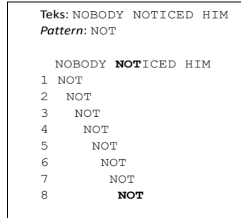
Gambar 2.2 Proses Pattern Matching dengan Algoritma Brute Force
