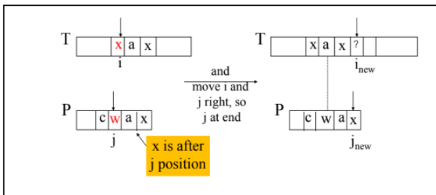
Gambar 2.5 Kasus Kemunculan x Terakhir Sudah Dilewati
