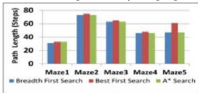
Gambar 4.3 Perbandingan Panjang Lintasan Ketiga Algoritma
