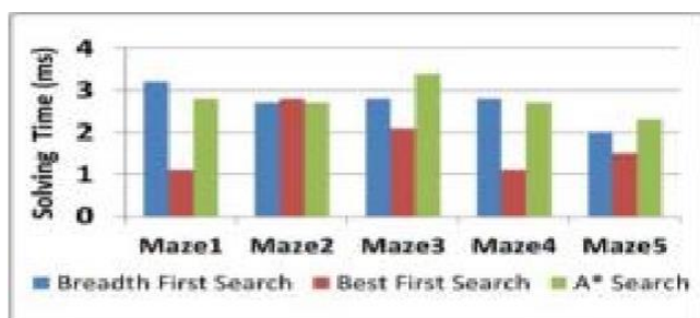
Gambar 4.2 Perbandingan Waktu Tempuh Ketiga Algoritma
