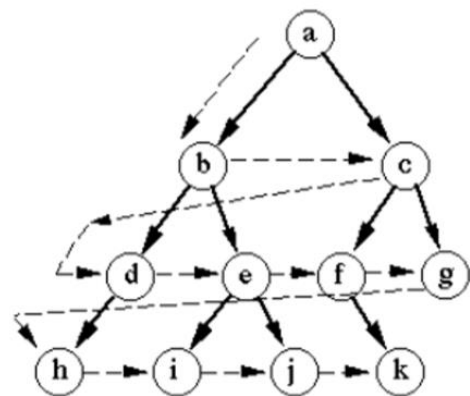
Gambar 2.1 Ilustrasi Algoritma Pencarian Melebar (BFS)
