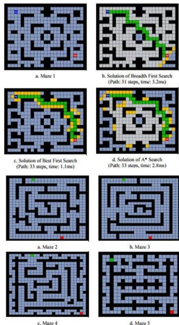
Gambar 4.1 Labirin Pengujian
