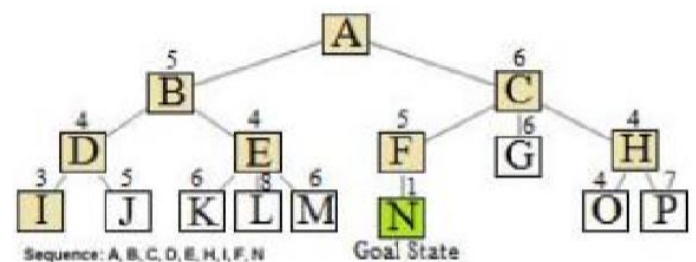
Gambar 2.3 Ilustrasi Algoritma A-Star(A*)
