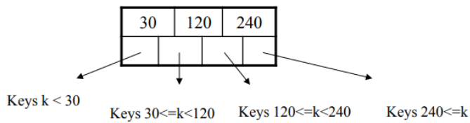
Gambar 3.1.1 Ilustrasi Simpul Dalam B+ Tree
