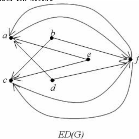
Gambar 2.17 Graf gabungan
