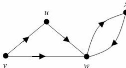
Gambar 2.18 Digraf
