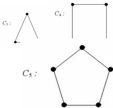
Gambar 2.12 Graf siklus
