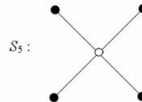
Gambar 2.14 Graf star
