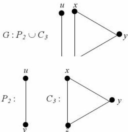
Gambar 2.17 Graf gabungan
