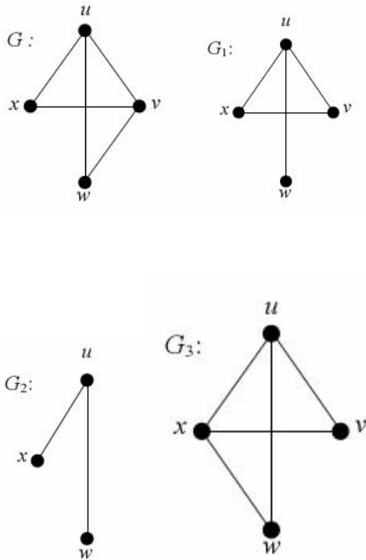
Gambar 2.6 Graf dan subgrafnya
