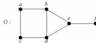
Gambar 2.9 Eksentrisitas
