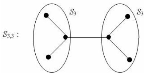
Gambar 2.16 Graf double star
