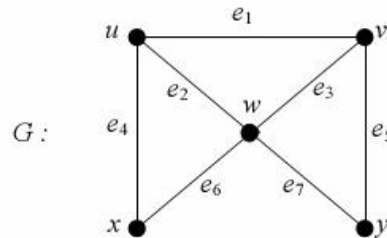
Gambar 2.5 Walk pada graf
