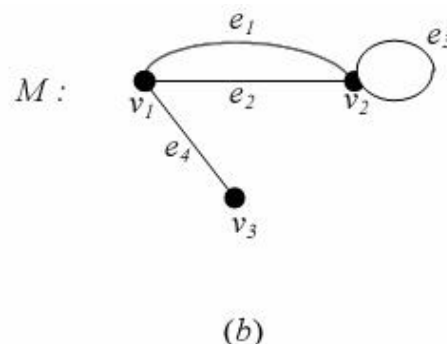
Gambar 2.1 Contoh graf
