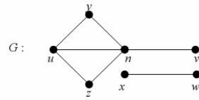
Gambar 2.8 Jarak pada graf
