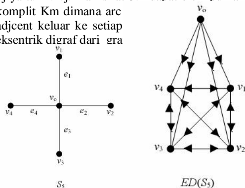
Gambar 3.1 Graf S_5 dan eksentrik digrafnya.
