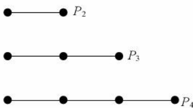
Gambar 2.11 Graf lintasan
