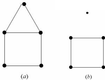
Gambar 2.7 Graf terhubung dan graf tak terhubung
