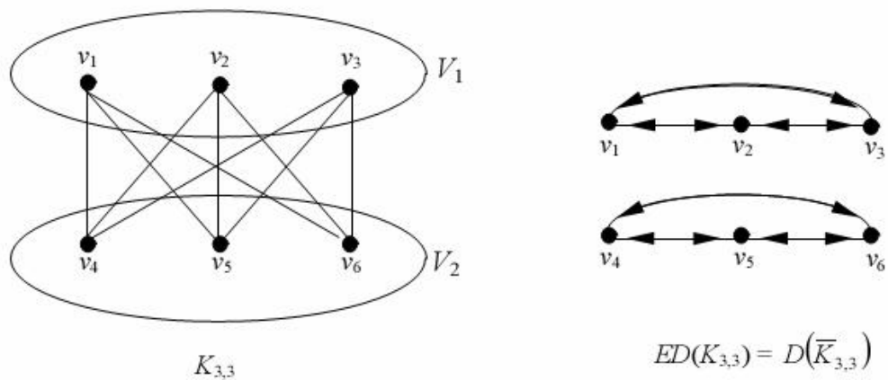
Gambar 3.3 Graf komplit bipartit K_{3,3} dan eksentrik digrafnya
