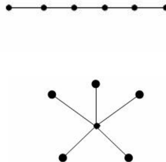
Gambar 2.15 Pohon
